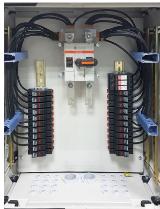
Низьковольтний пристрій для моніторингу блоків сонячних фотогальванічних модулів – шафа збору потужності SC-SP/11-24
