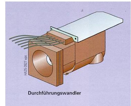
проходной трансформатор
