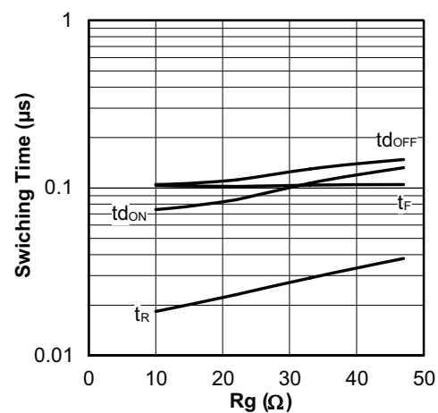
Fig. 12 - Typical Switching Time vs. R_G T_J = 125\text{ }^\circ\text{C} ; L = 200\text{ }\mu\text{H} ; V_{CE} = 300\text{ V} ; I_{CE} = 20\text{ A} ; V_{GE} = 15\text{ V}
