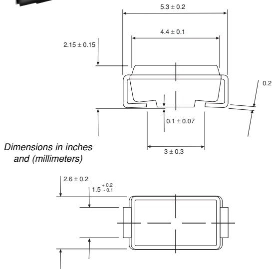
DO-214AC (SMA)
