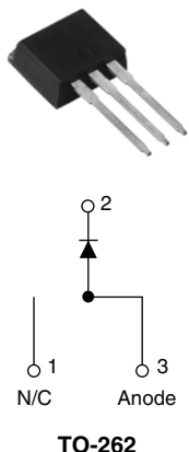
VS-15ETX06-1PbF
