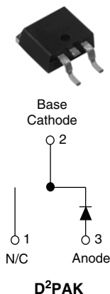
VS-15ETX06SPbF
