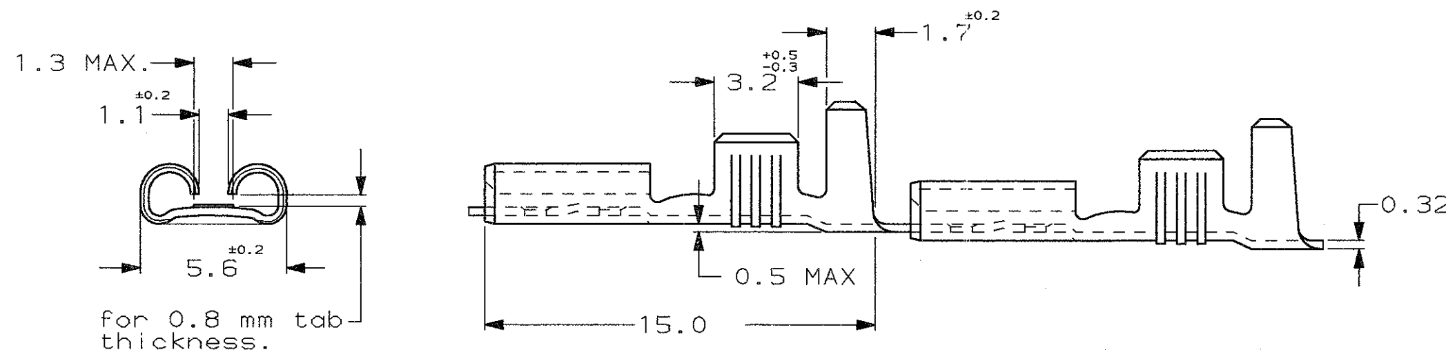
SEZIONE A-A (SECTION A-A)
