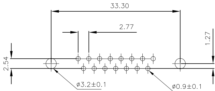
P.C.B. LAYOUT
