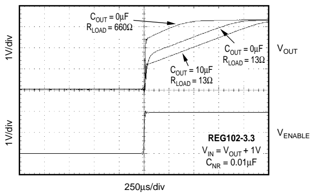
TURN-ON
