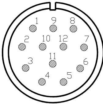
Pinning encoder (male)
