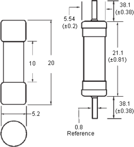
Dimensions : Millimetres
