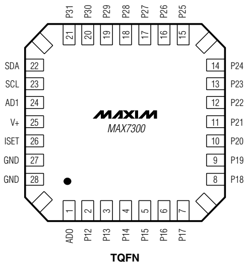
TQFN
