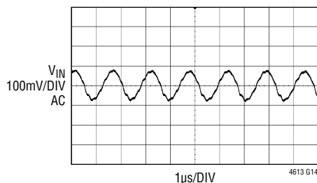
Input Ripple
