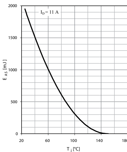
Fig. 9 Avalanche energy
