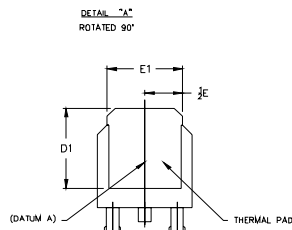
VIEW A-A
