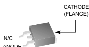
JEDEC TO-263AB
