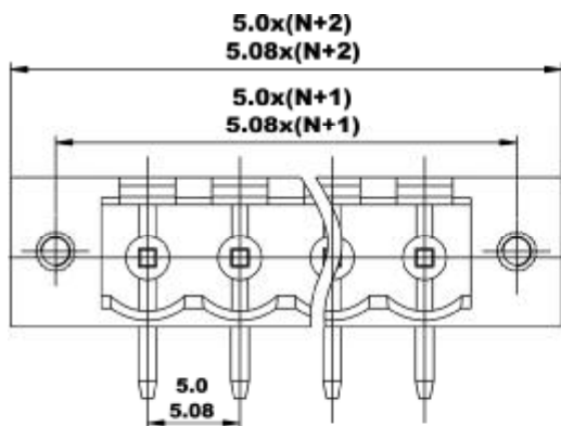
2EDGRM-5.0 2EDGRM-5.08
