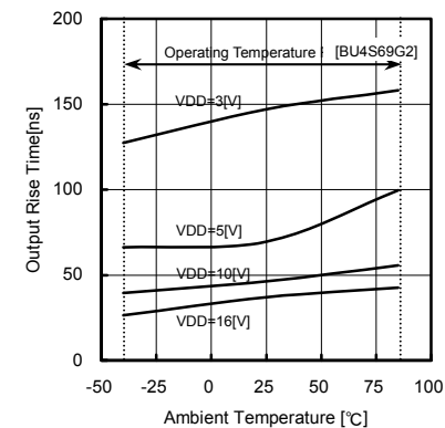
Fig.24 Output rising time tTLH
