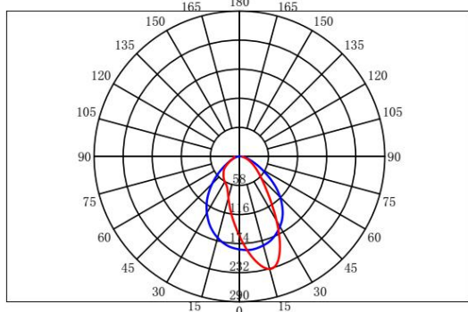
配光曲线
