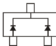
BAT54C
