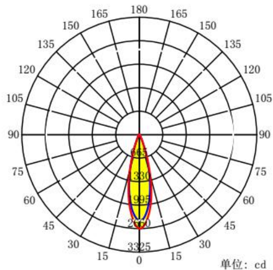
配光曲线
