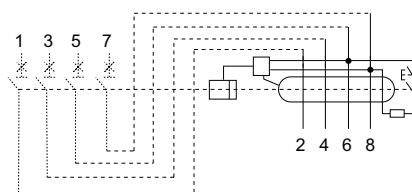
Схема соединения
