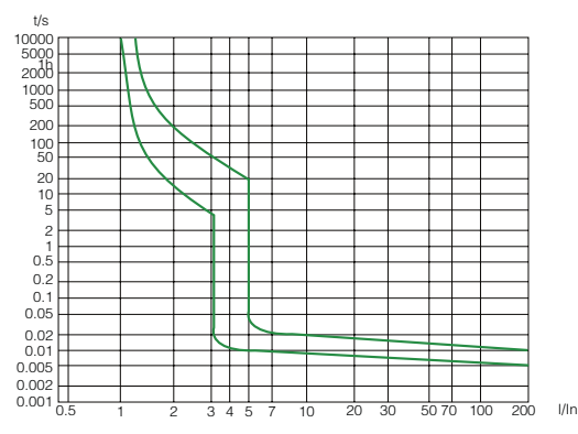
Характеристика В
