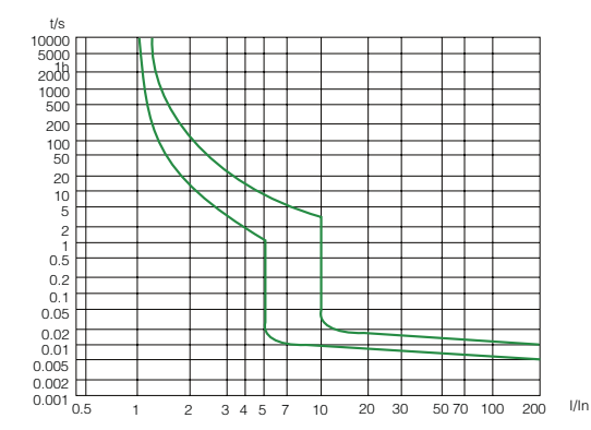
Характеристика С
