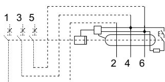
Схема соединения
