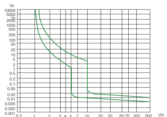
Характеристика С
