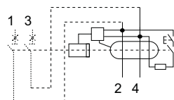
Схема соединения
