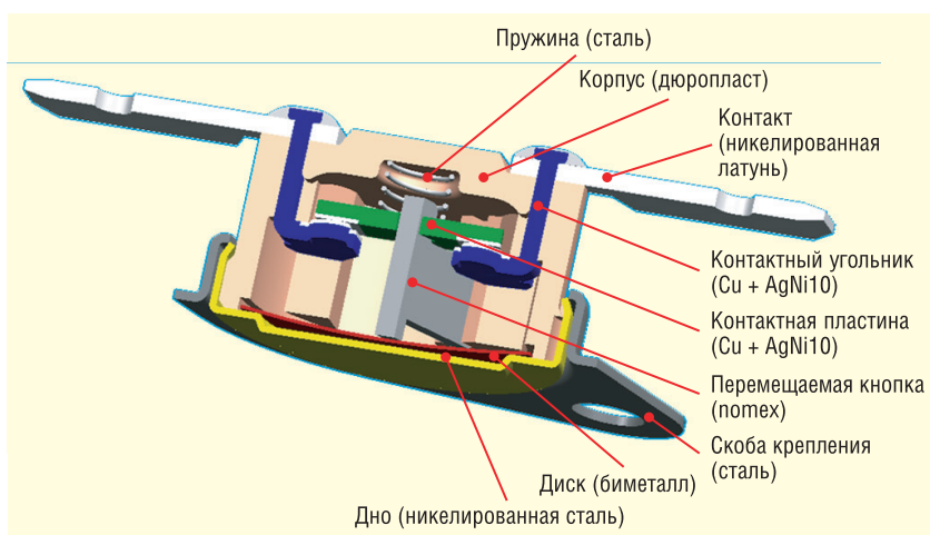
Рис. 1. Конструкция термовыключателя MICROTHERM CZ серии R
