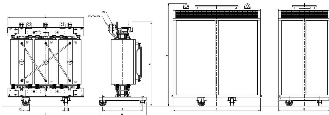
Trasformatore IP00 - Transformator IP00 - Transformer IP00
